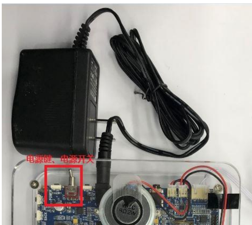
整体接线图
